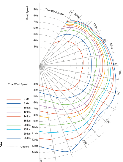
Polar Diagram Polaire de vitesse Deep draft and Classic rig
